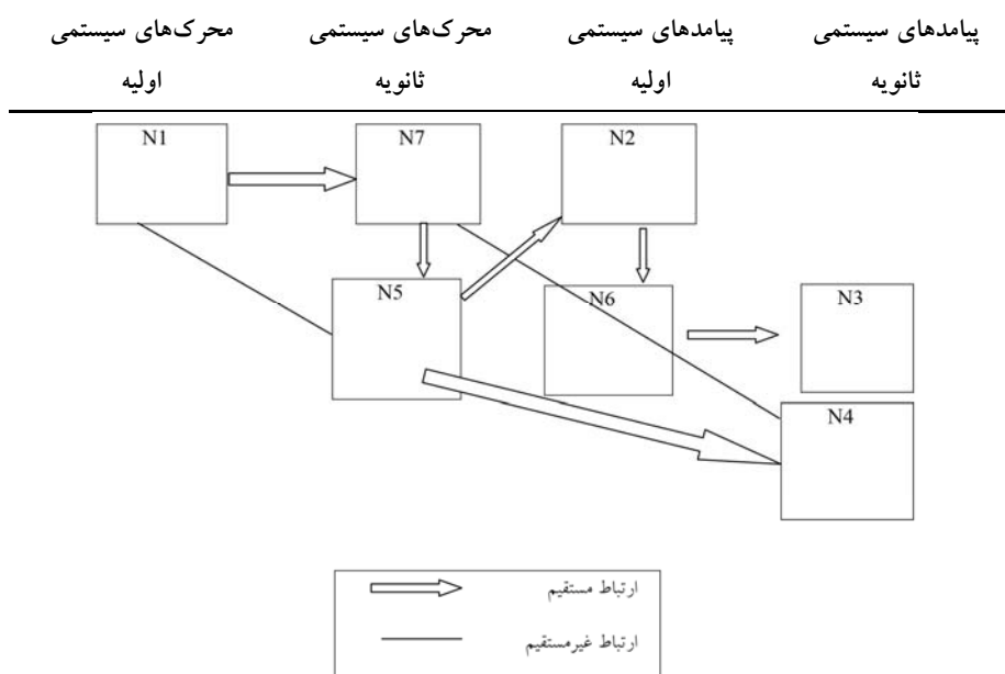
شکل ۲. نمونه نمودار SID بر مبنای داده‌های نمودار پیشین IRD
